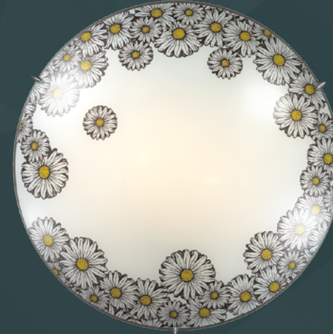
арт. 2215 Ø 300mm | 100mm E27 2x60W
